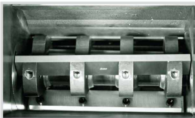
Paddle Blade (SG-30&SG-36)
